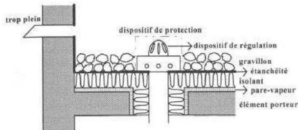
Exemple de constitution d'une toiture terrasse stockante
