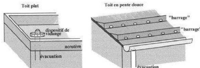
Principe de stockage d'eau en toiture d'après (STU, 1982b)
