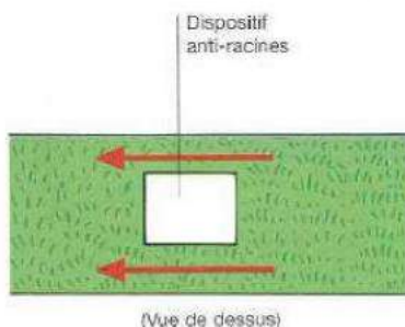
Réalisation d'une tranchée avec arbre et dispositif anti-racine Source CETE du Sud-Ouest
