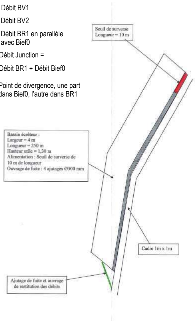
Figure 29 : Localisation des ouvrages hydrauliques projetés
