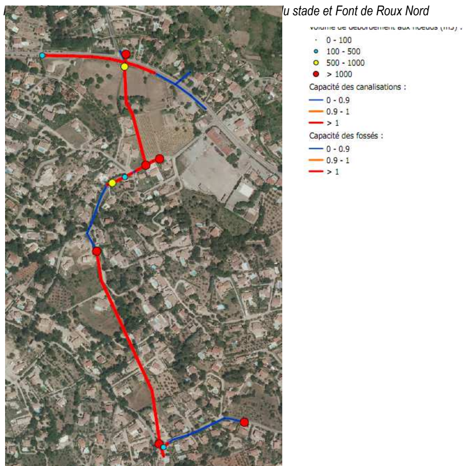
Figure 27 : Insuffisance réseau chemin du stade et Font de Roux Nord
