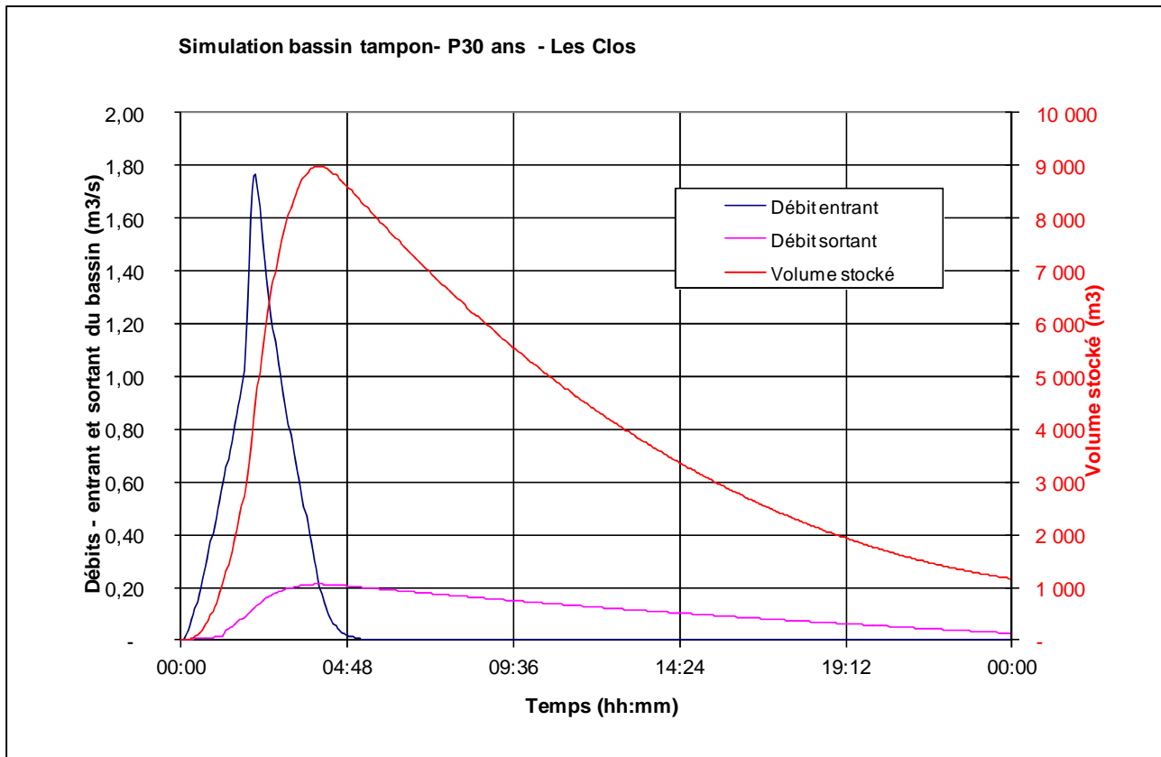
Figure 14 : Hydrogramme pour la crue simulée – secteur les Clos
