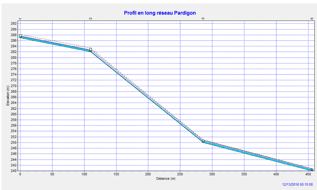
Figure 34 : Profil en long de la future collecte des eaux pluviales – quartier Pardigon
